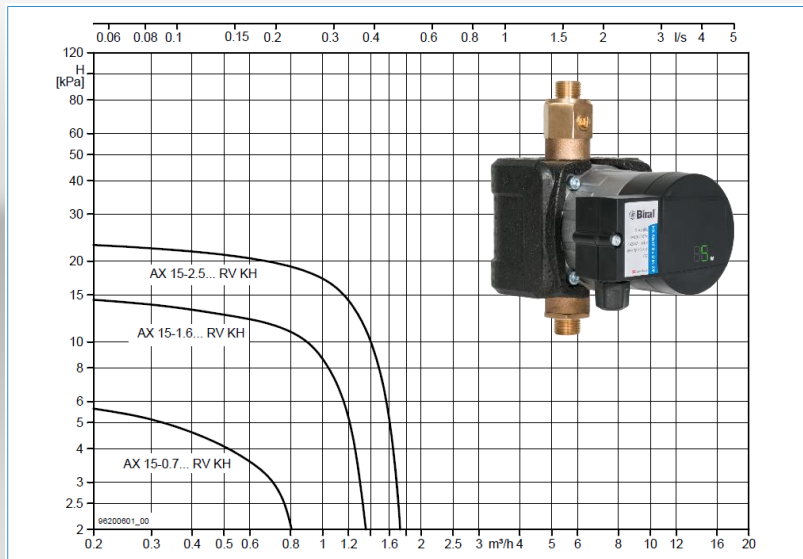
Curve caratteristiche – AX 15 BLUE
